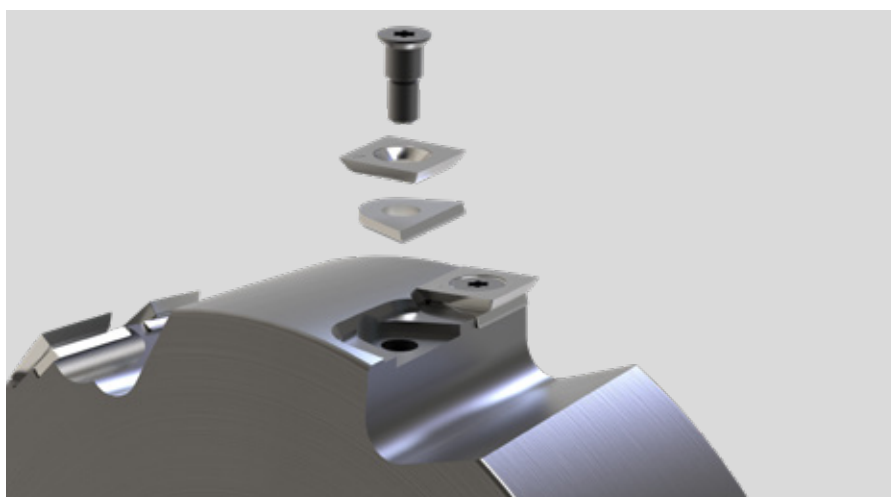
A késbefogó robbantott ábrája, beleértve a kopásvédő lemezt
