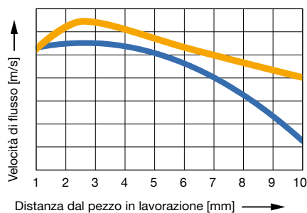
Velocità di flusso in funzione della distanza dal pezzo
